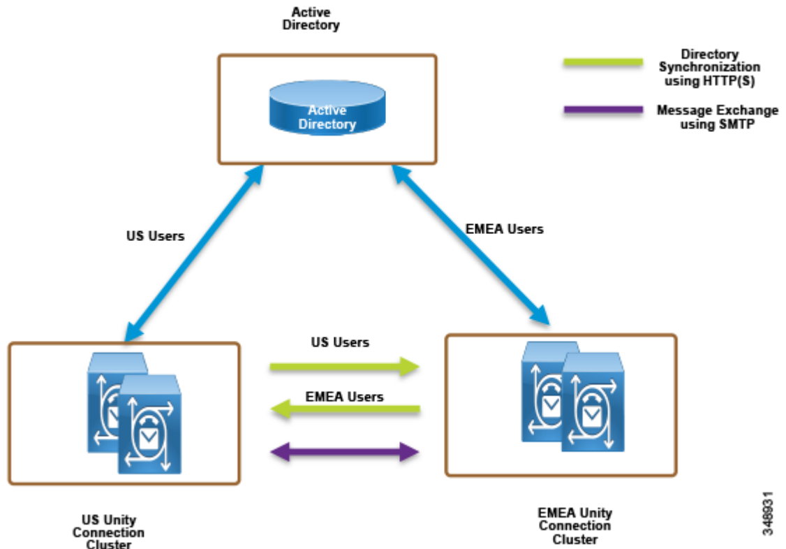
図 5-4 2 つの Unity Connection クラスターの HTTPS インターネットワーキング
