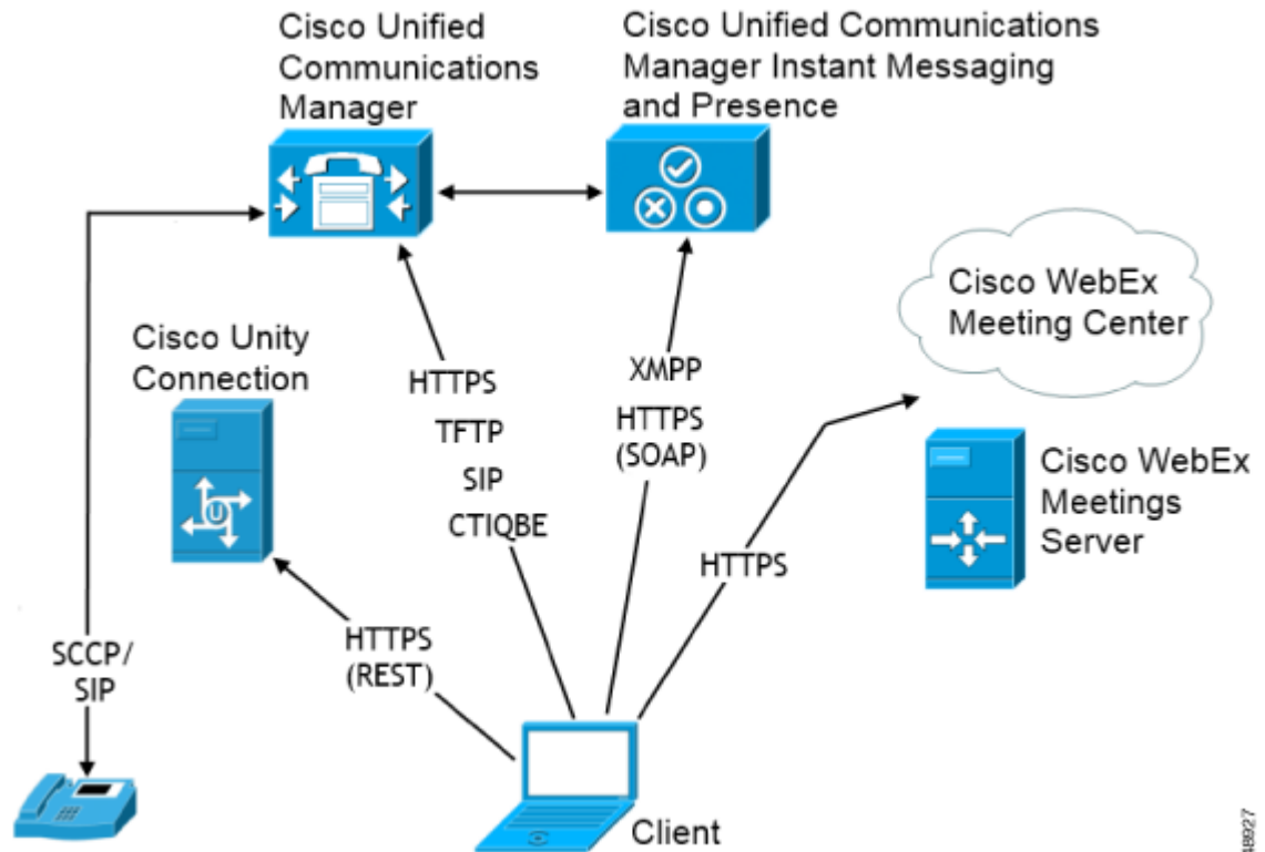
図 2-5 Cisco Unified Communications IM and Presence のアーキテクチャ
