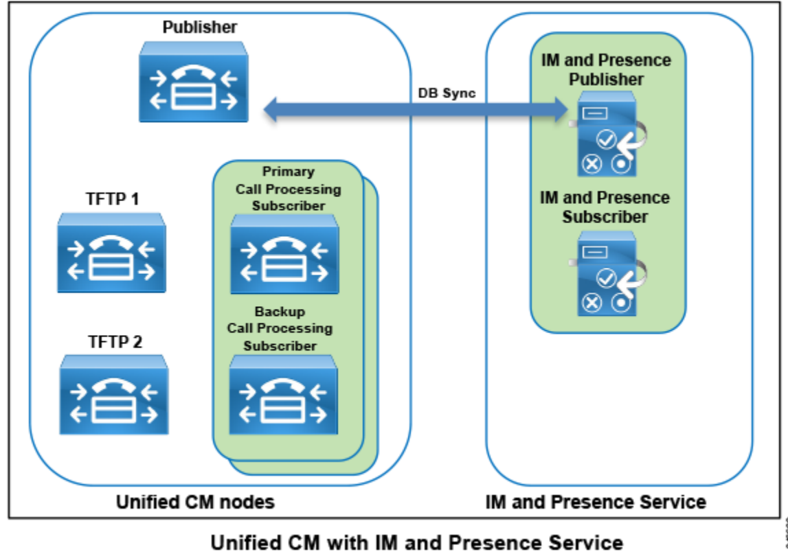
図 2-4 Unified CM and IM and Presence Service クラスターの展開
