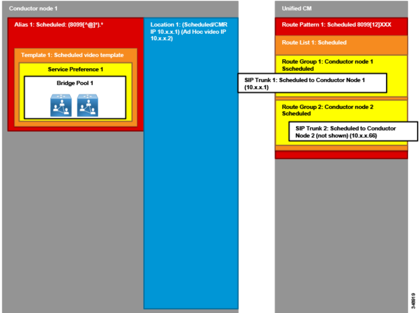
図 3-20 Unified CM CMR およびスケジュール済み会議
