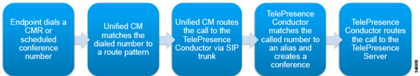
図 3-7 無期限またはスケジュール済み会議のコールフロー
