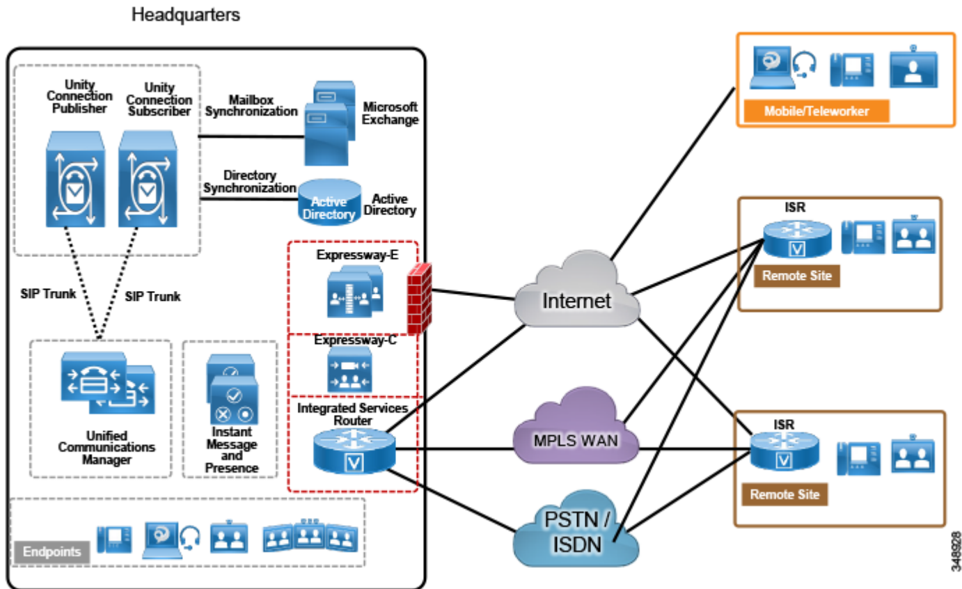
図 5-1 アーキテクチャの概要
