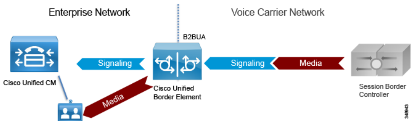
図 4-13 IP PSTN アーキテクチャ
