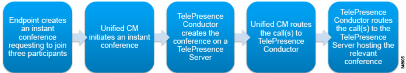
図 3-6 インスタント会議のコールフロー
