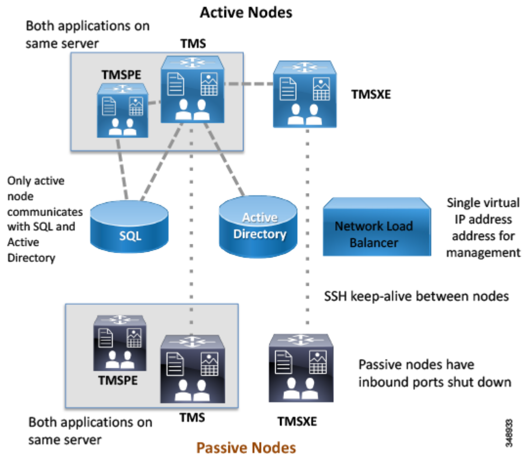
図 5-5 アーキテクチャの概要
