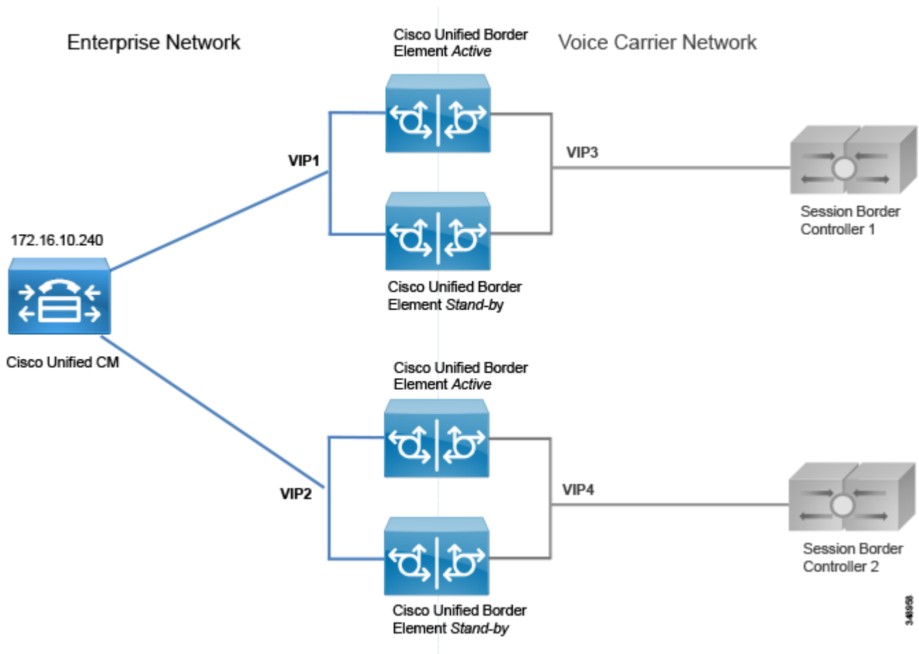
図 4-25 別々の SBC に接続された複数の Cisco Unified Border Element
