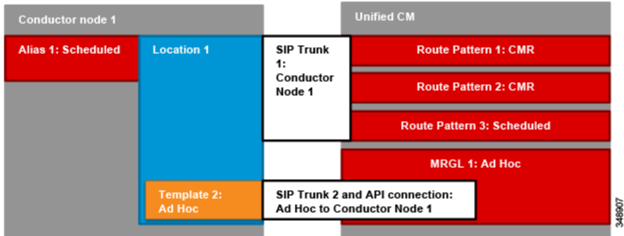
図 3-8 Unified CM と TelePresence Conductor 間の API および SIP トランク接続
