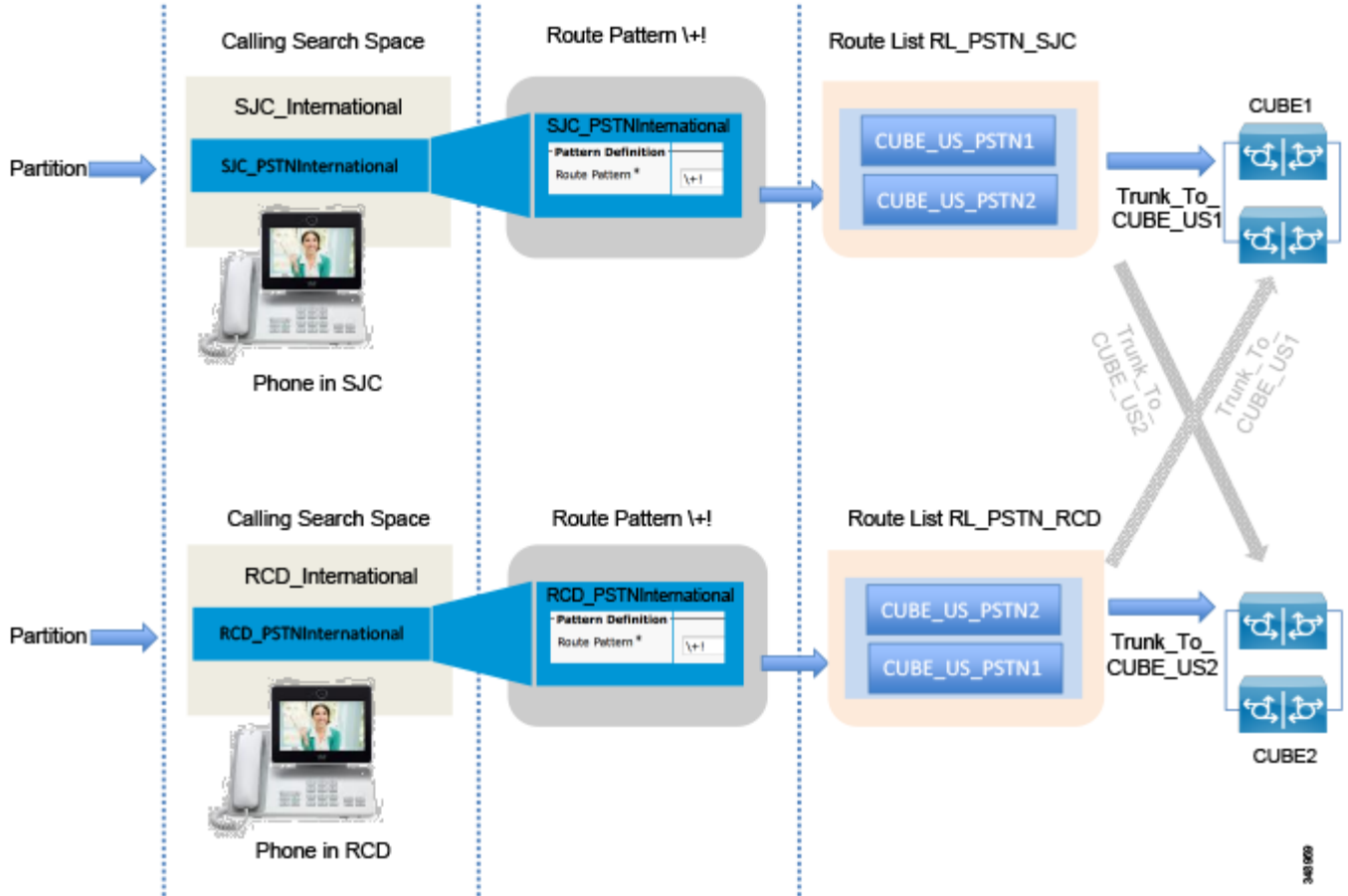
図 4-26 Cisco Unified Border Element 接続用の Unified CM の設定
