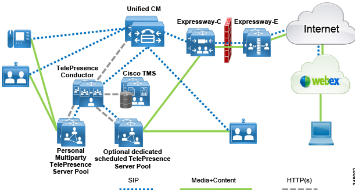
図 3-2 標準的な展開
