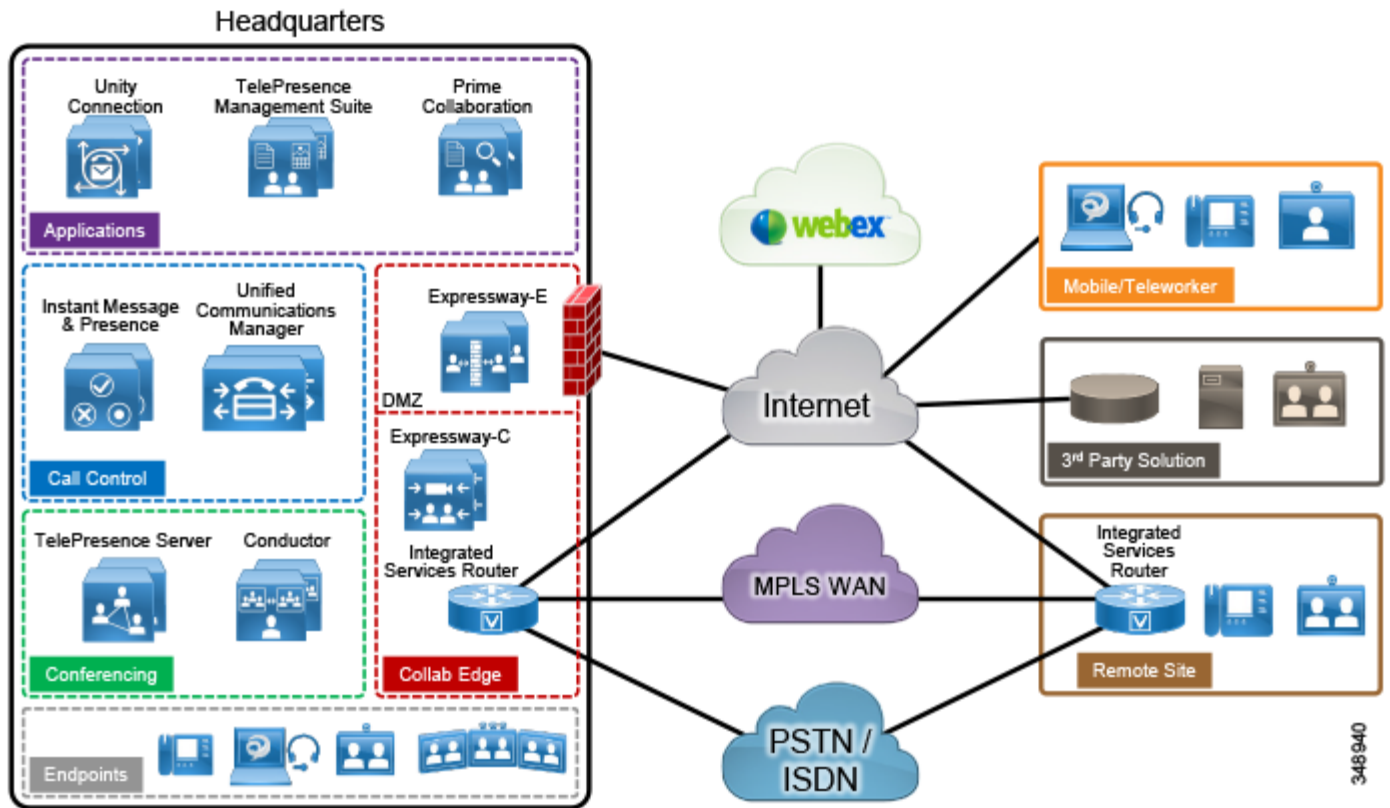
図 1-1 エンタープライズ コラボレーション向けシスコ推奨アーキテクチャ
