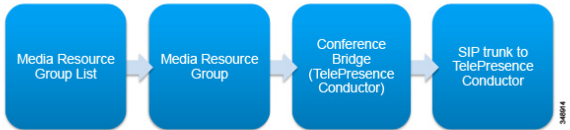
図 3-15 インスタント会議用の Unified CM の内部設定フロー
