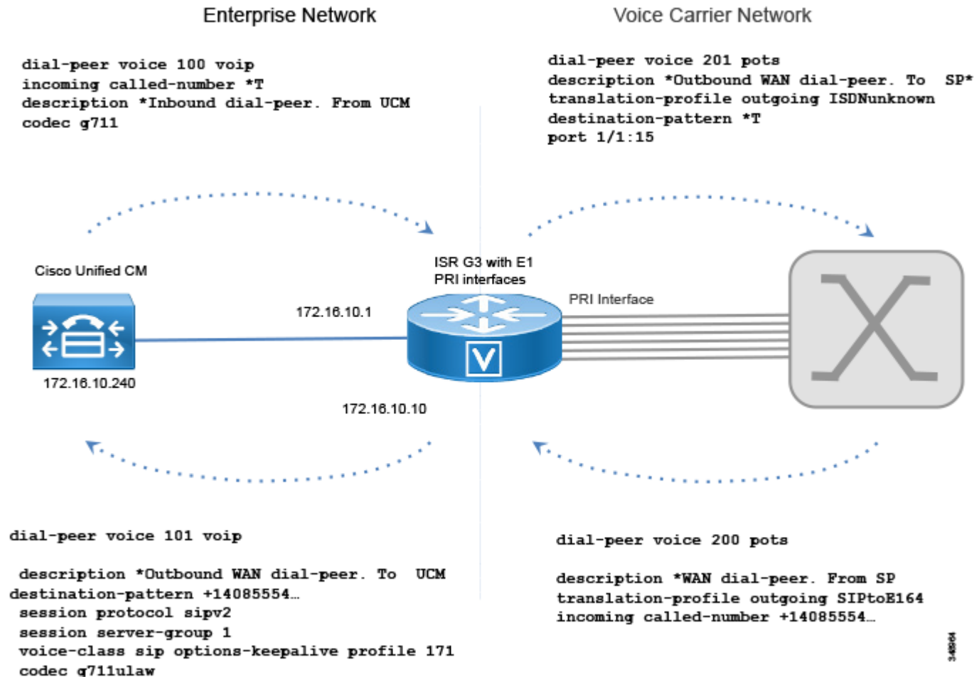
図 4-31 音声ゲートウェイのダイヤルピア設定
