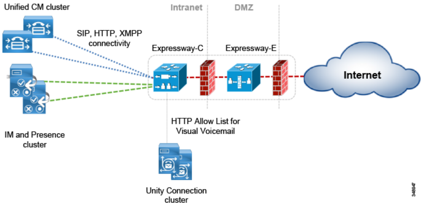
図 4-8 Unified CM、IM and Presence サービス、および Unity Connection への Expressway 接続
