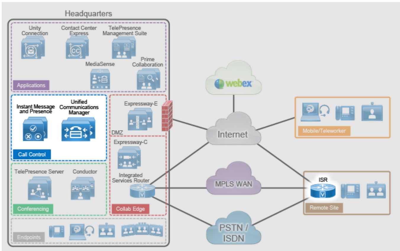
図 2-1 プリファード アーキテクチャの概要
