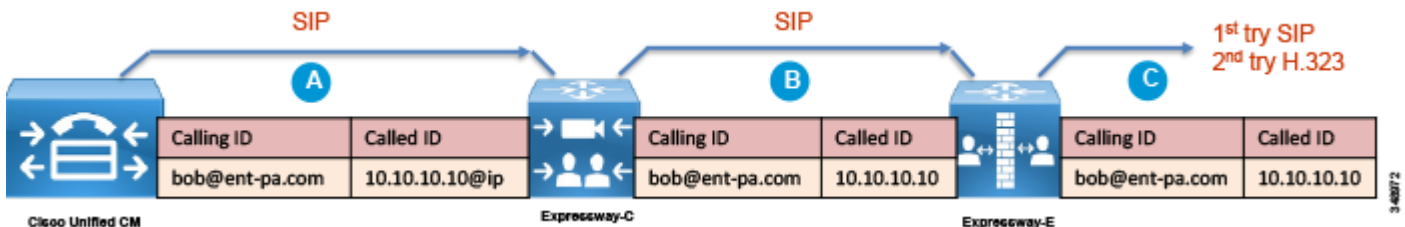
図 4-11 アウトバウンド IP ベース ダイヤリングの例
