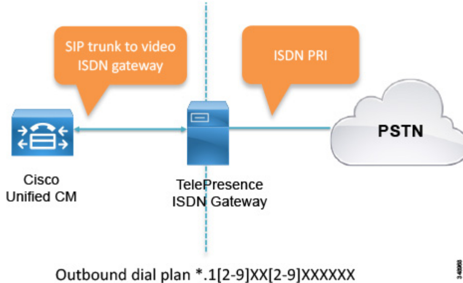
図 4-15 ビデオ ISDN ゲートウェイダイヤルプラン
