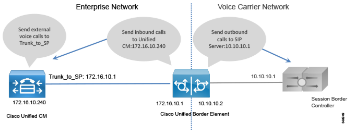
図 4-14 Cisco Unified Border Element のトランキングに関する留意点
