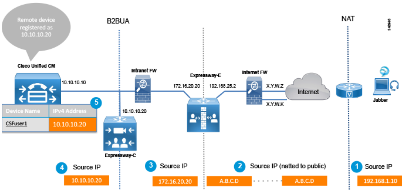
図 4-7 パケットの寿命に基づく NAT
