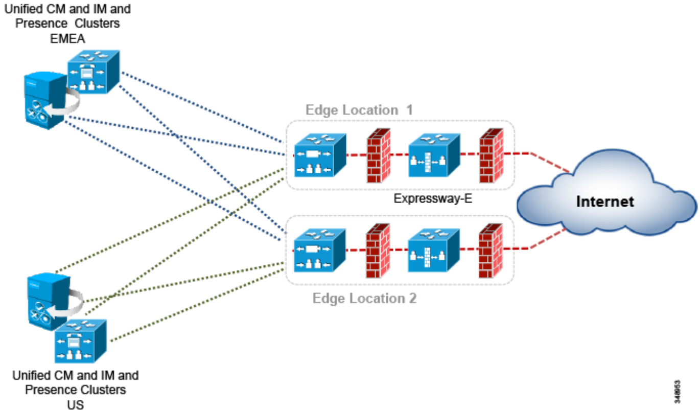
図 4-19 複数の Unified CM および IM and Presence クラスタのサービス検出
