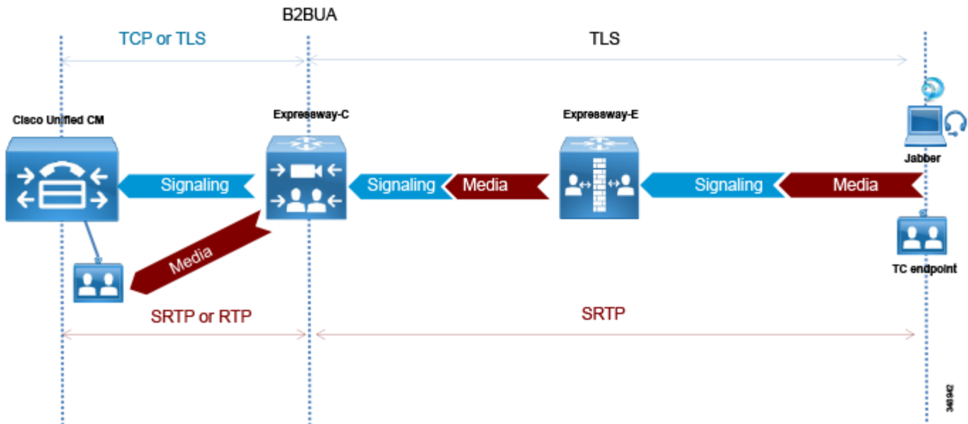
図 4-2 Expressway 上の B2BUA とコール レッグ
