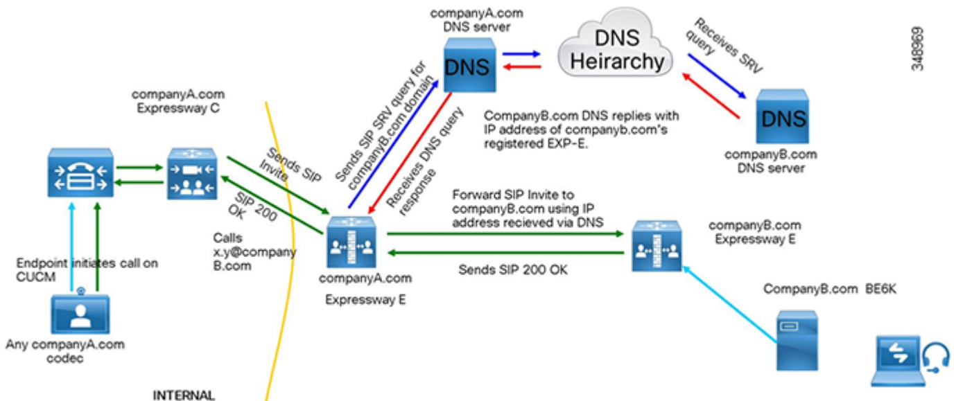
図 4-10 DNS を使用した URI ダイアリング
