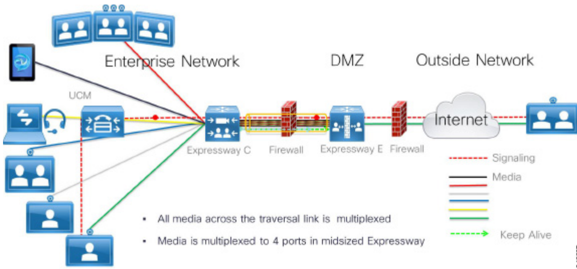
図 4-3 Expressway-C の多重化とキープアライブ
