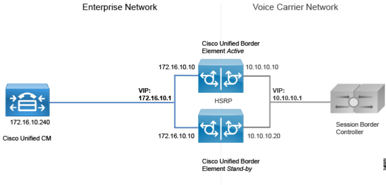
図 4-17 Cisco Unified Border Element のボックスツーボックス冗長性
