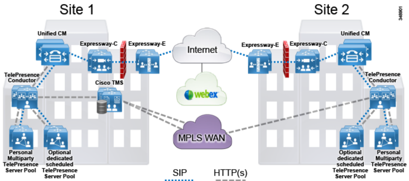
図 3-1 アーキテクチャの概要
