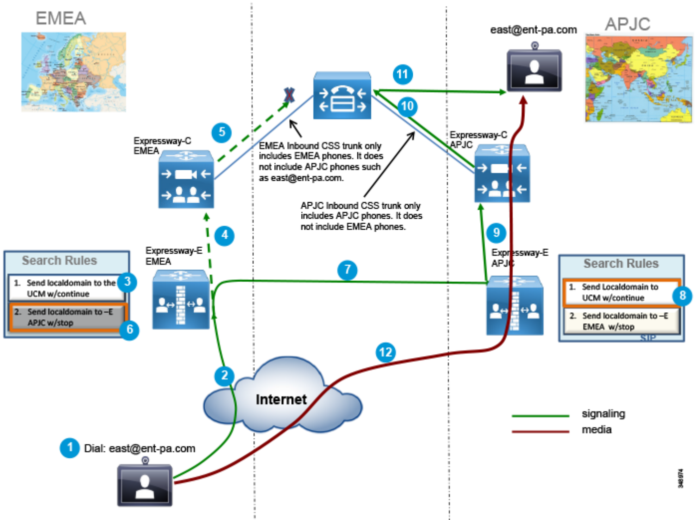
図 4-22 宛先に最も近い Expressway クラスタの選択
