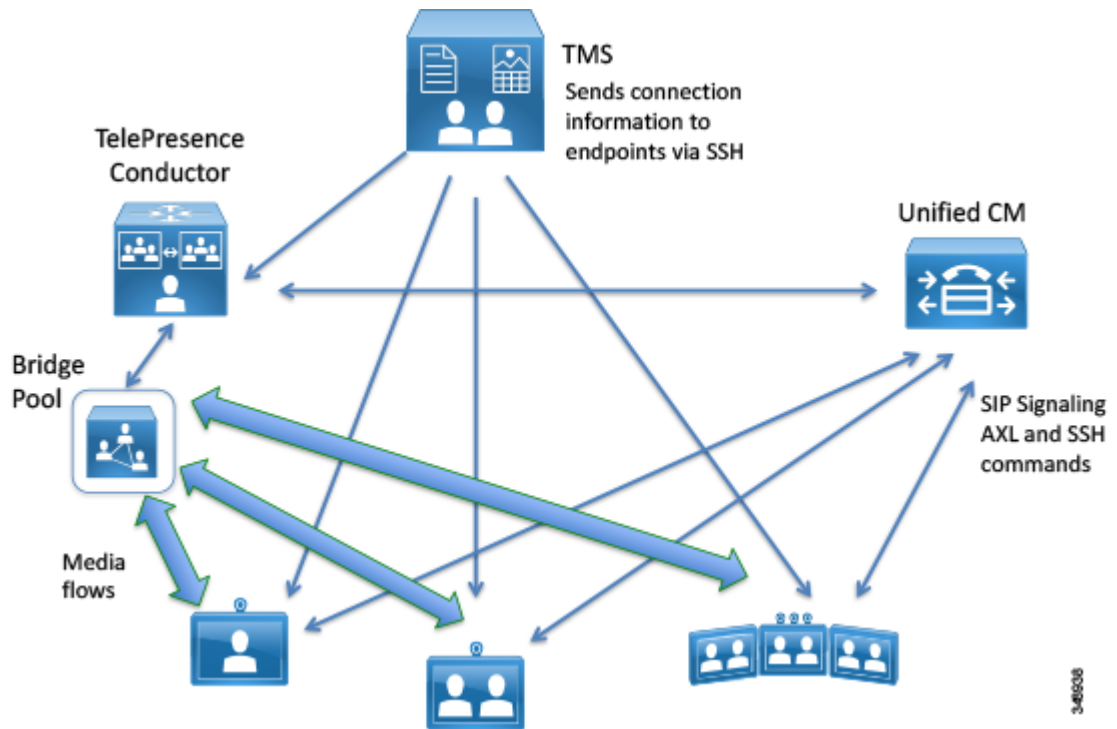
図 5-10 Cisco TMS と Unified CM 管理対象エンドポイントの直接通信
