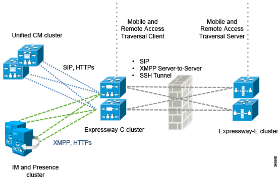
図 4-16 Expressway サービス接続
