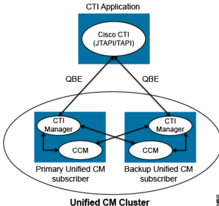
図 2-3 CTI のアーキテクチャ
