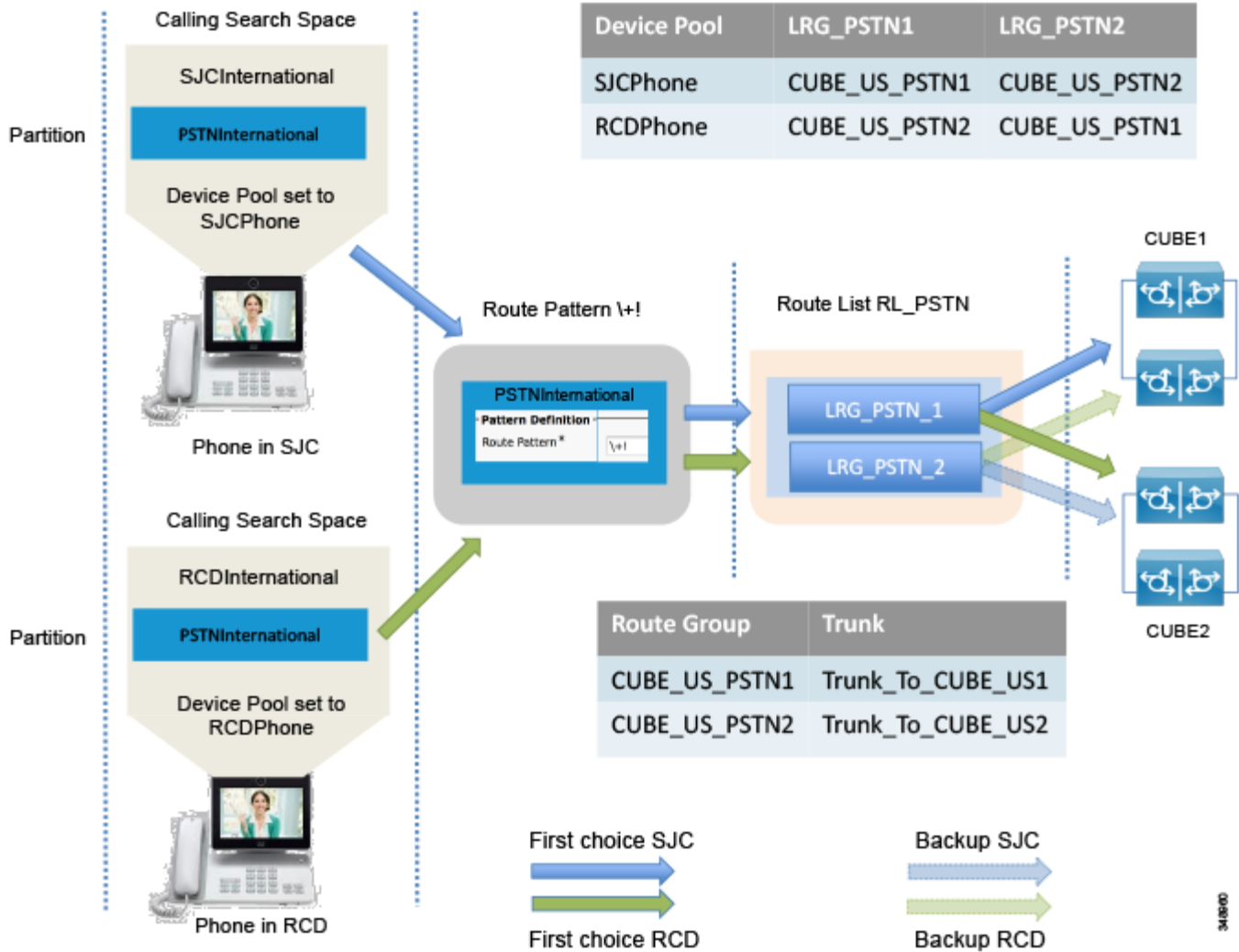
図 4-27 ローカル ルート グループ アプローチを使用した Cisco Unified Border Element 接続用の Unified CM の設定
