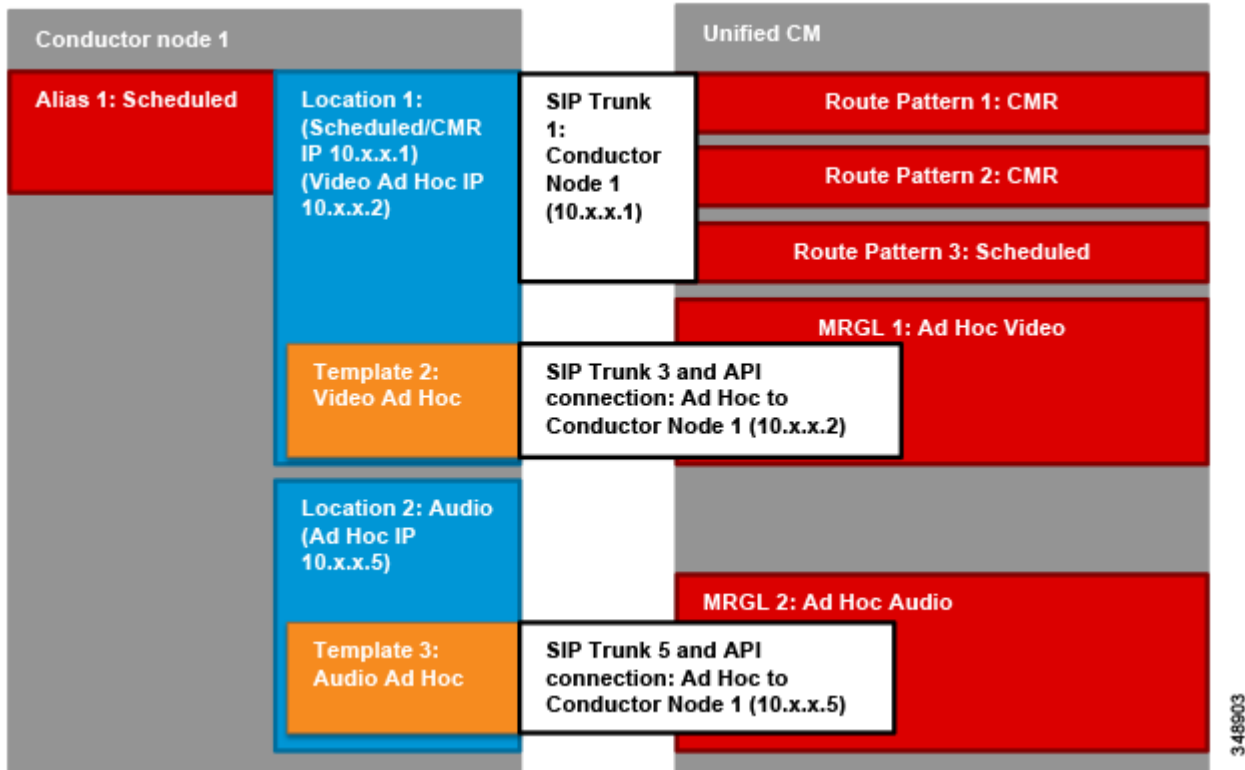
図 3-3 Unified CM および TelePresence Conductor SIP トランク
