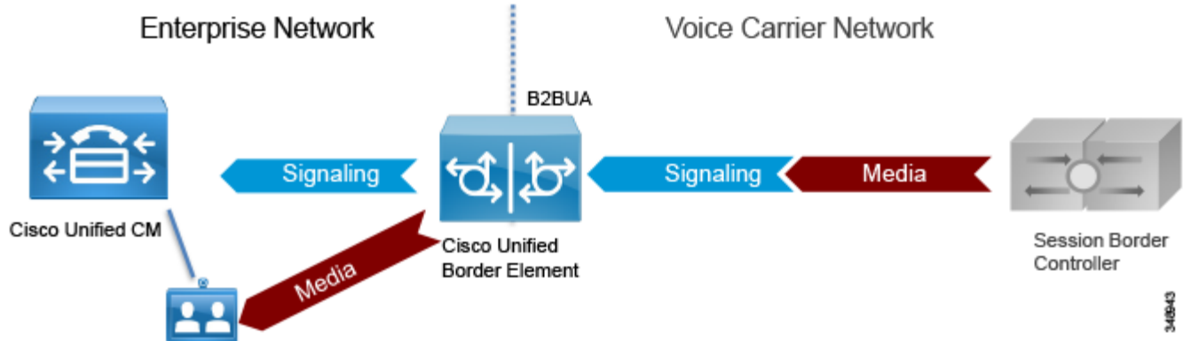
図 4-4 B2BUA としての Cisco Unified Border Element
