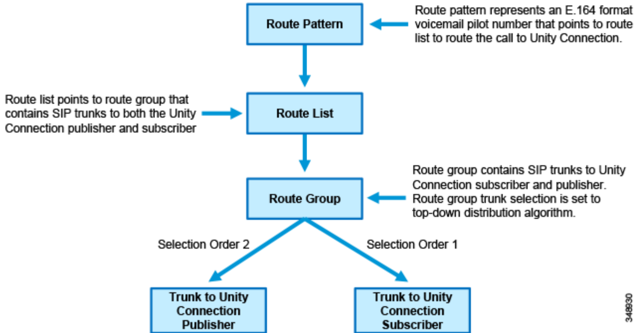
図 5-3 Unity Connection SIP トランクの選択
