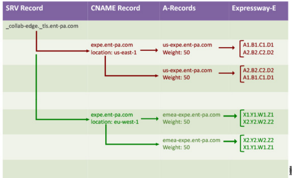
図 4-20 遅延ベース ルーティング用 Route 53 DNS レコード構造
