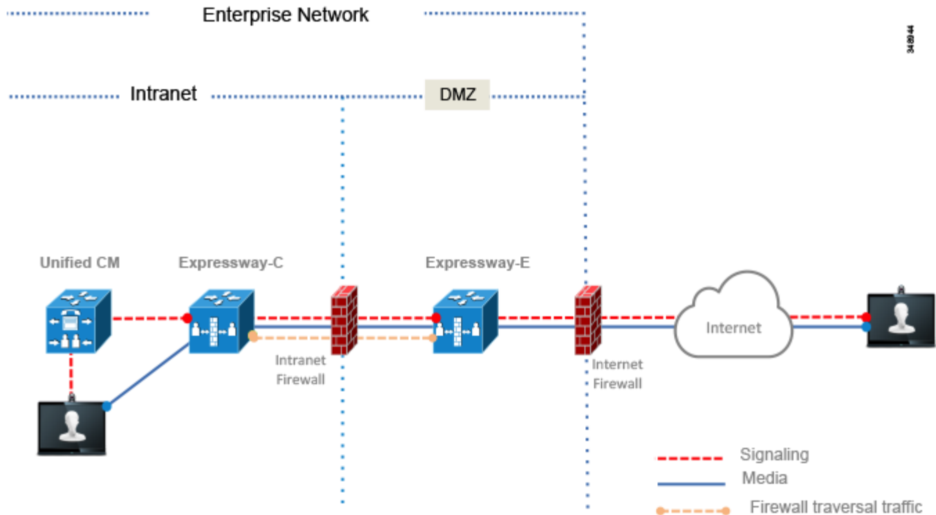
図 4-5 Expressway-C と Expressway-E のファイアウォールトラバースルプロセス
