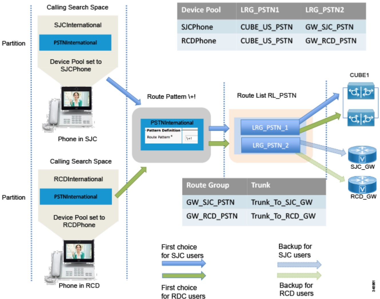
図 4-28 ローカル ISDN ゲートウェイを使用した集中型 PSTN アクセスに関する設定
