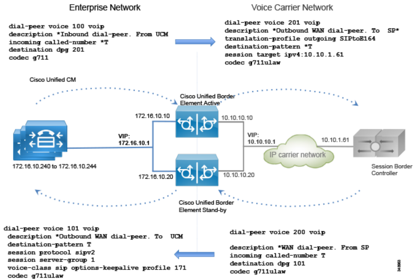
図 4-30 Cisco Unified Border Element のダイヤルピア設定
