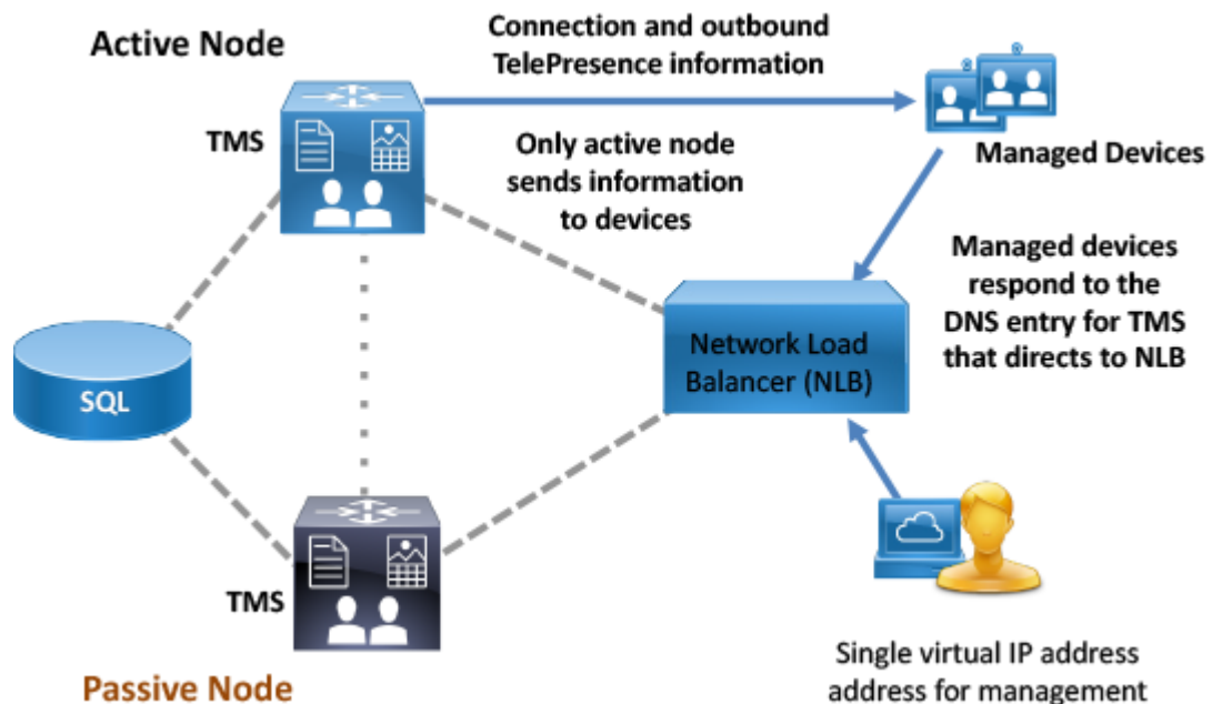
図 5-8 NLB による管理対象デバイスからアクティブ TMS ノードへの通信の指示
