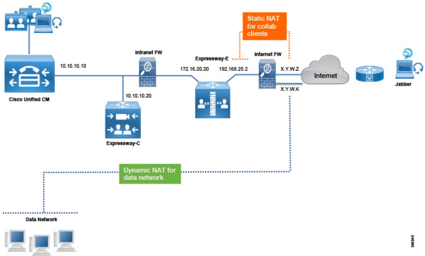
図 4-6 インターネット ファイアウォール上の NAT インターフェイス
