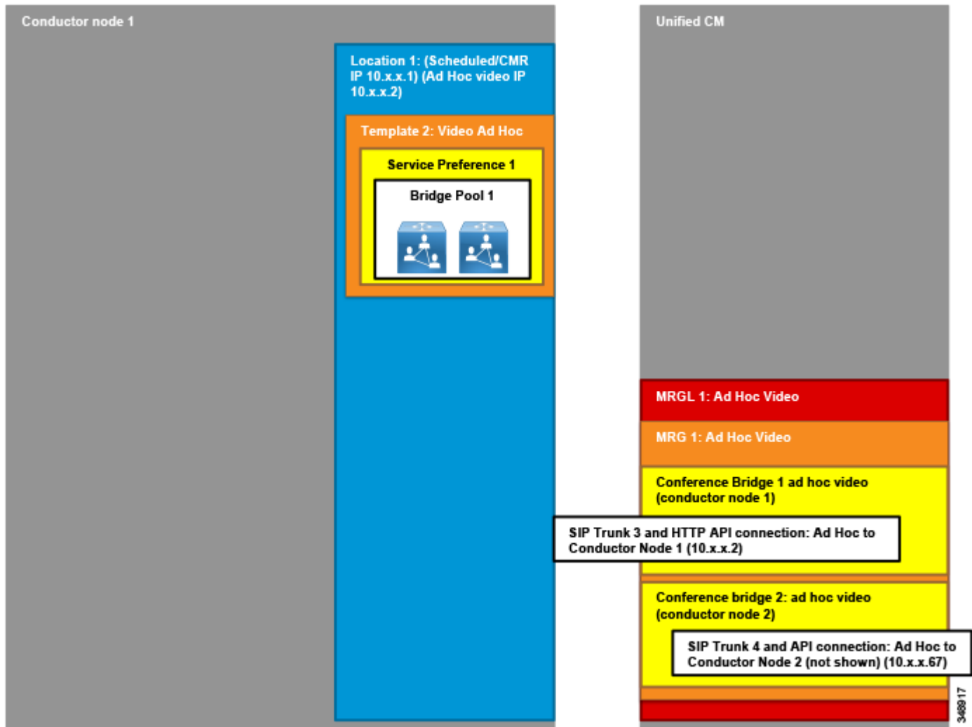
図 3-18 Unified CM インスタント構成
