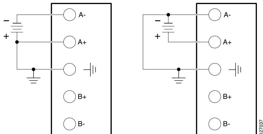
図 4 1つの電源のみに接続 — 電源 A または電源 B
