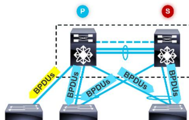
Com peer-switch o domínio vPC é visto como um switch único no STP
