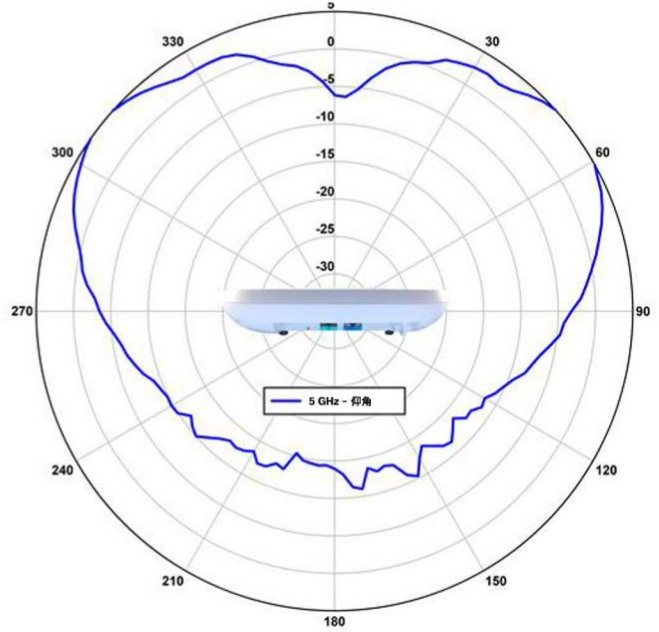
思科 C9130AXI 天线方向图 5 GHz - 仰角 - 单频天线元件
