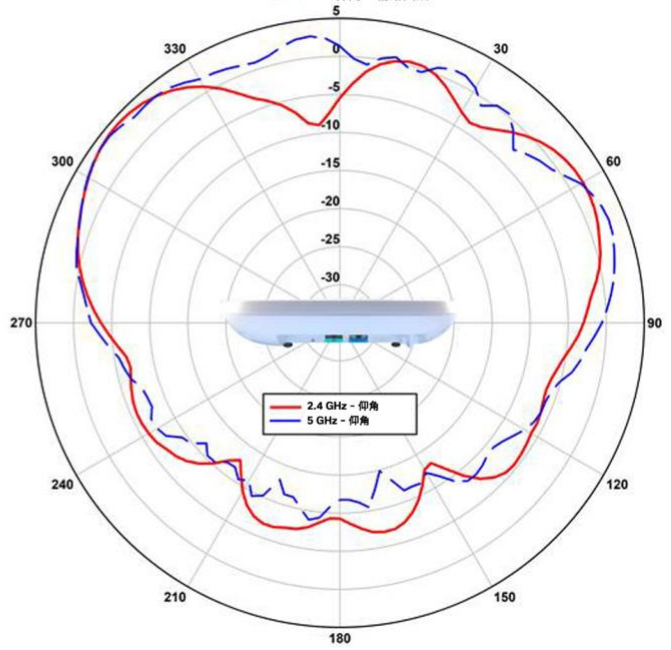
思科 C9130AXI 天线方向图 2.4 & 5 GHz - 仰角 - 辅助天线
